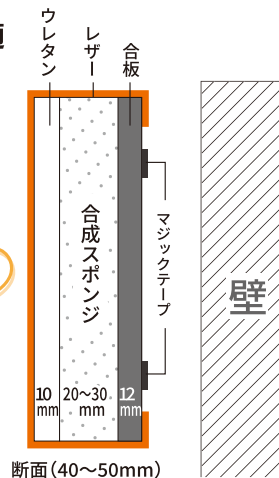
断面(40~50mm)
