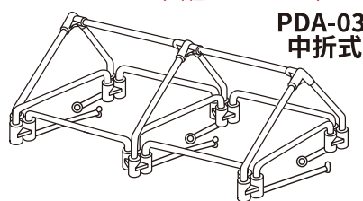
PDAテント骨組図 (20パーツ)
